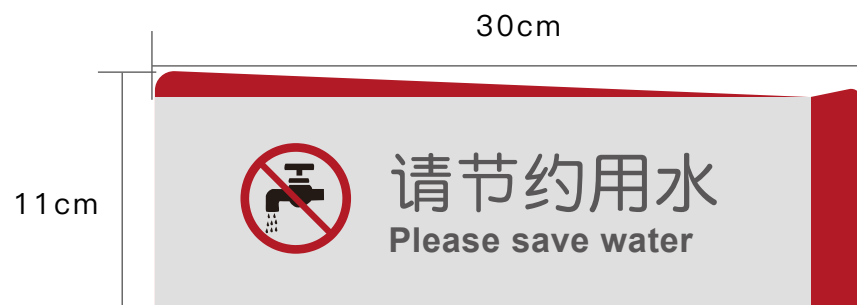
正视图
